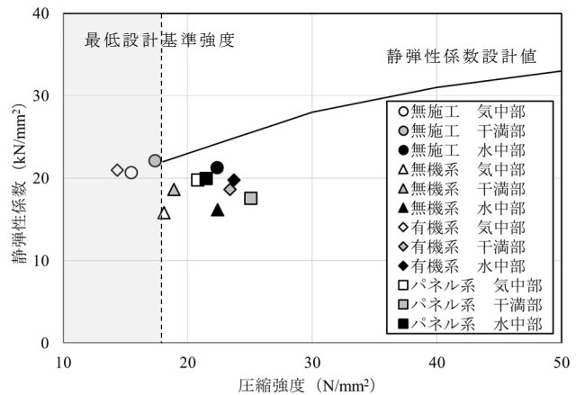
Fig. 3 圧縮強度および静弾性係数の測定結果 Compressive strength and static elastic modulus
