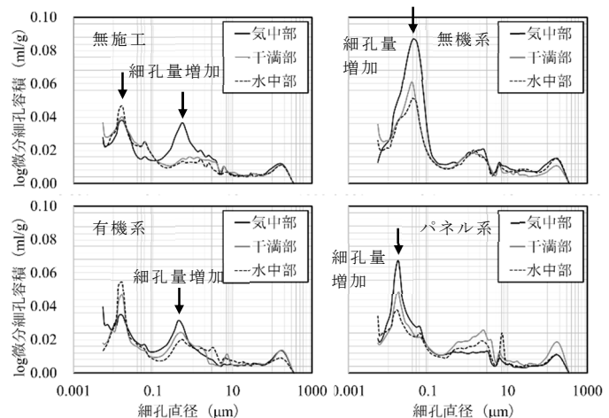
Fig. 5 細孔径分布の測定結果 Pore size distribution
